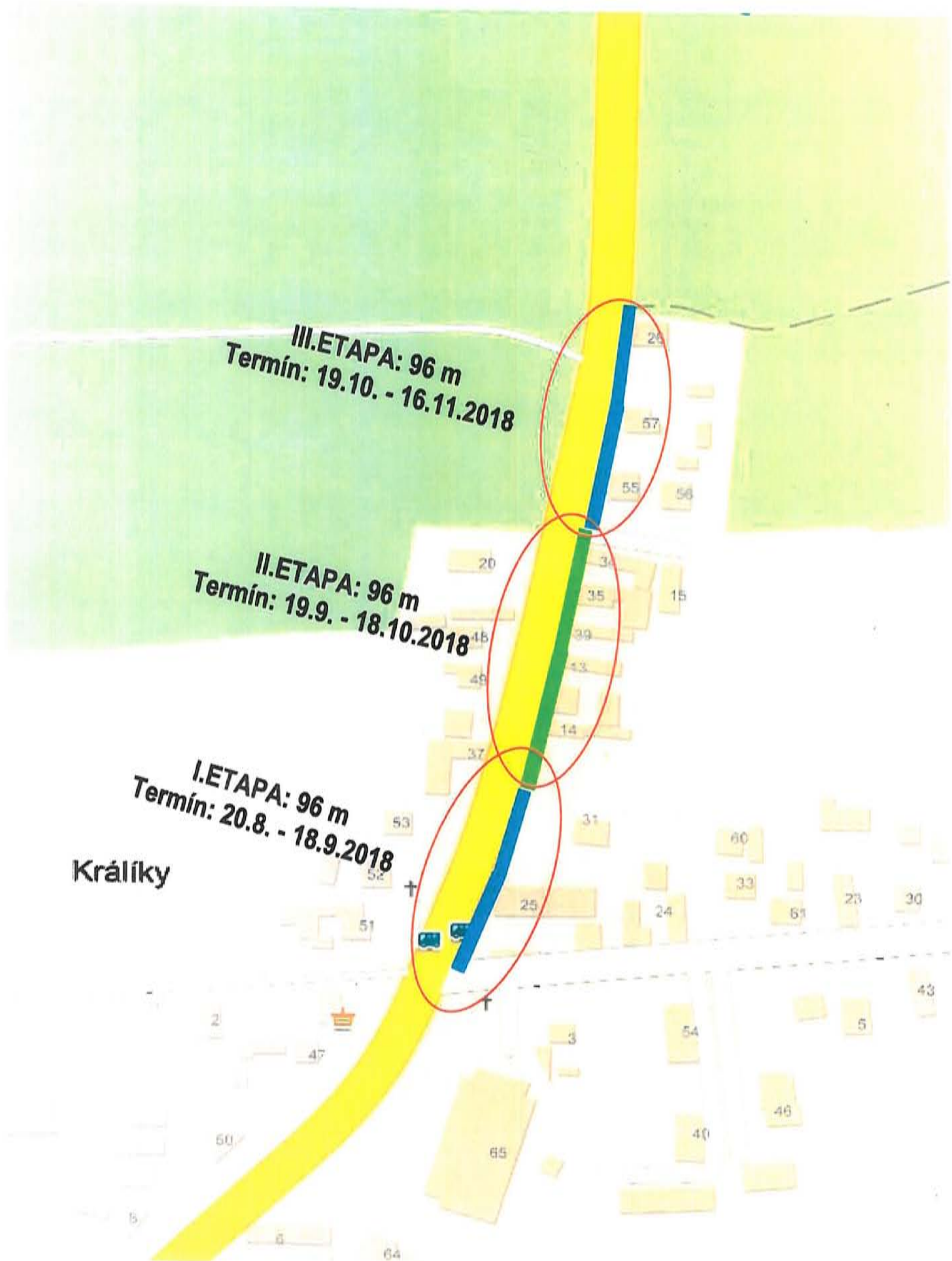
DOPRAVNÍ OPATŘENÍ NA SILNICI II/326 V OBCI KRÁLÍKY REKONSTRUKCE VODOVODNÍHO ŘADU V TERMÍNU: 20.8. - 16.11.2018 STAVBA ROZDĚLENA NA 3. ETAPY
